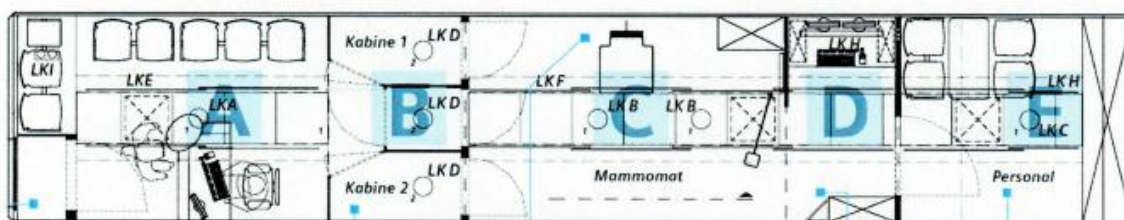
Rys. Schemat poglądowy zabudowy naczepy
